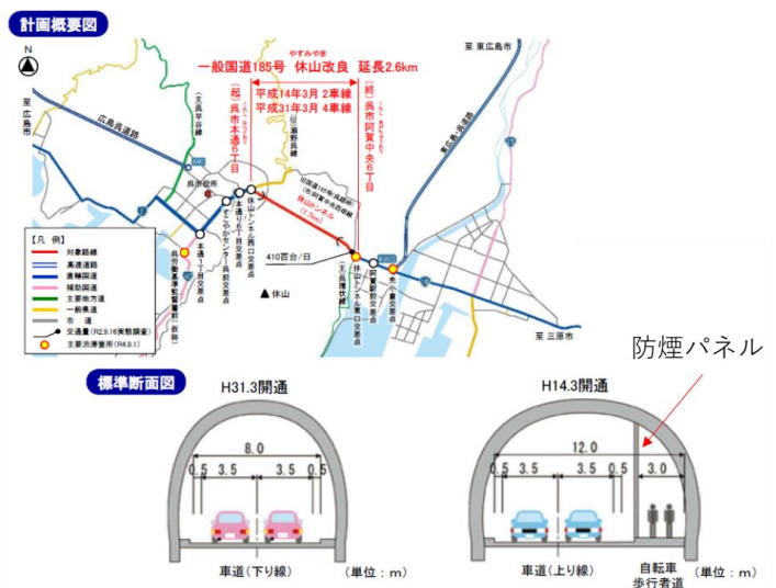
図-18 一般国道185号 休山改良（休山トンネル） （出典：事後評価結果（令和5年度））
